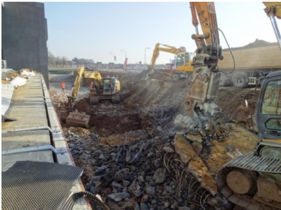
Figuur 90: Sloop van de betonnen overkluizing
