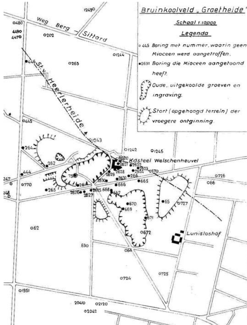
Figuur 275: Boring in het bruinkoolveld Graetheide in 1917
