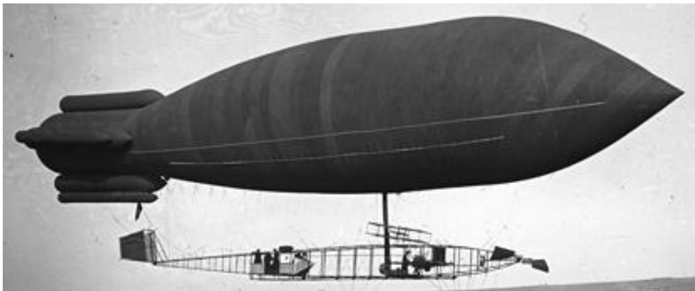
Figuur 259: Vliegtuigframe onder een zeppelin om die te kunnen besturen
