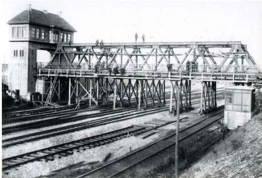
Figuur 371: IJzeren brug in aanbouw, deze geeft toegang tot Bergerweg in 1930 (het poortgebouw is het nieuwe seinhuis met uitzicht over het rangeerterrein)
