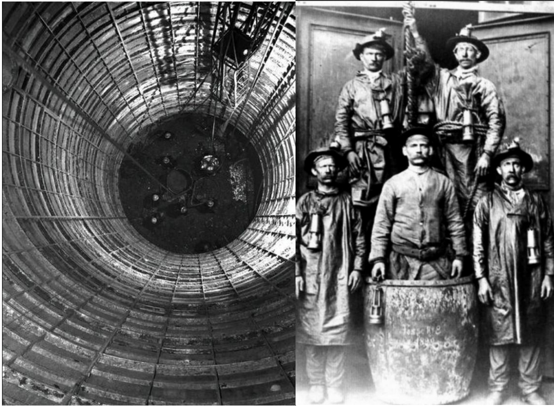
Figuur 250: Afdiepen van de schacht met schop en houweel; de mannen worden in de zandbak vervoerd
