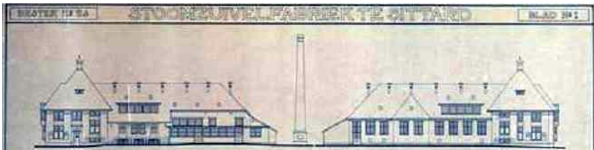
Figuur 221: Ontwerp van architect Wielders voor de melkfabriek in 1913
