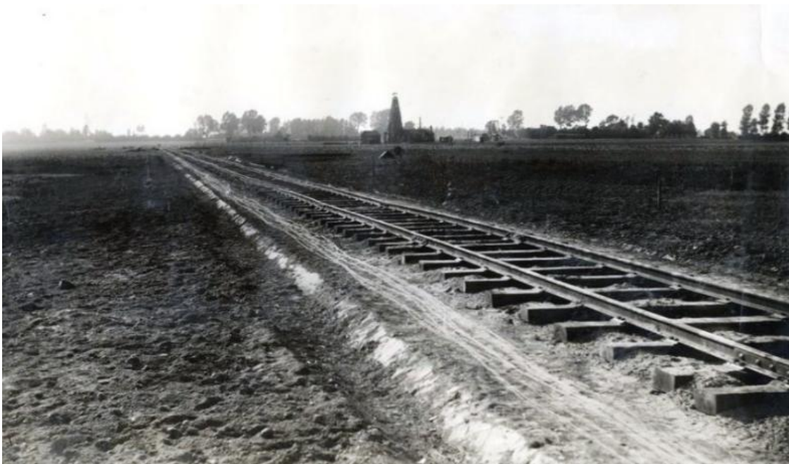
Figuur 251: Aanleg mijn Maurits - spoor van de boortoren naar het Station Lutterade 1916
