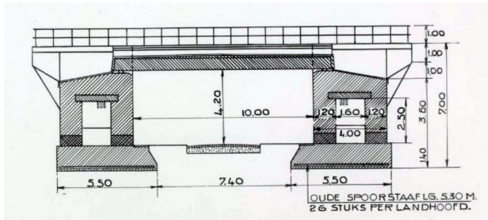
Figuur 368: Afmetingen van de spoortunnel, gefundeerd op oude spoorrails
