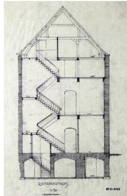
Figuur 14: Bouwtekening Kritzraedthuis uit 1620
