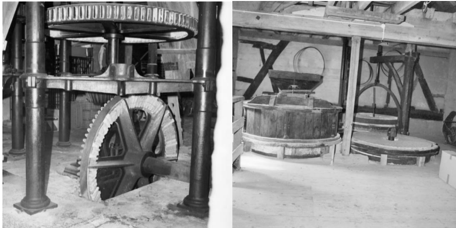
Figuur 139: Binnenwerk van de Ophovenmolen, links de aandrijf-as van het waterrad, rechts de molenstenen
