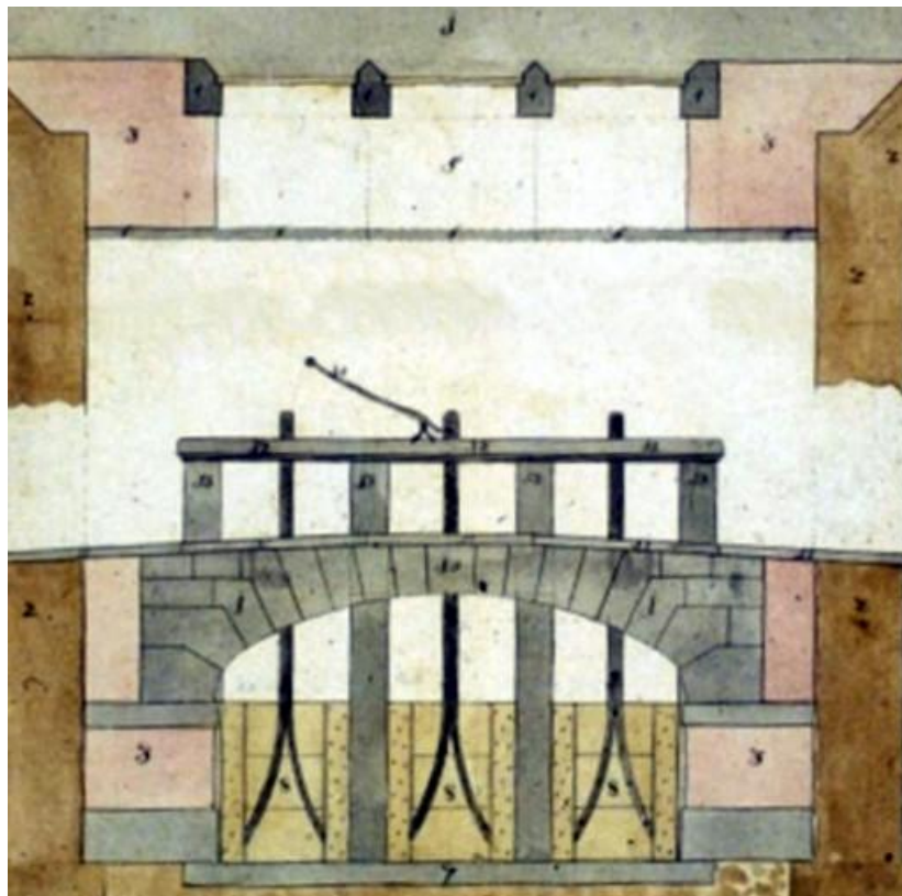
Figuur 172: Bouwtekening van de nieuwe Stenen Sluis uit 1752
