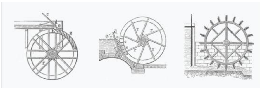
Figuur 133: bovenslagrad
