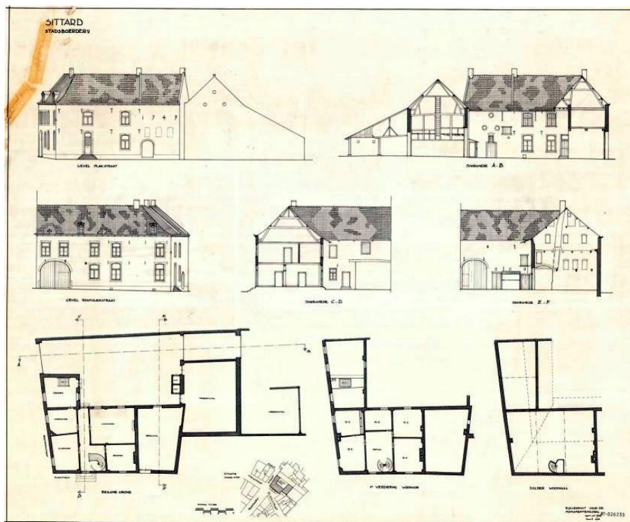
Figuur 151: Bouwtekening van de Stadsboerderij, waar nu de grote winkel van V&D staat
