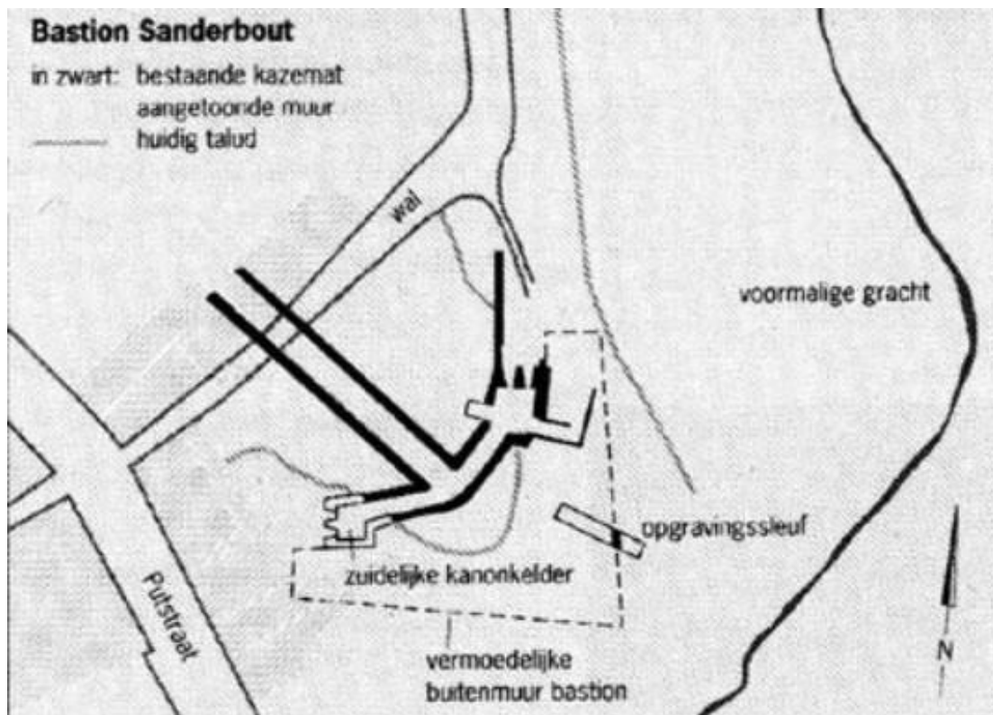
Figuur 259: Plattegrond fort Sanderbout met ondergrondse gang onder de wal door
