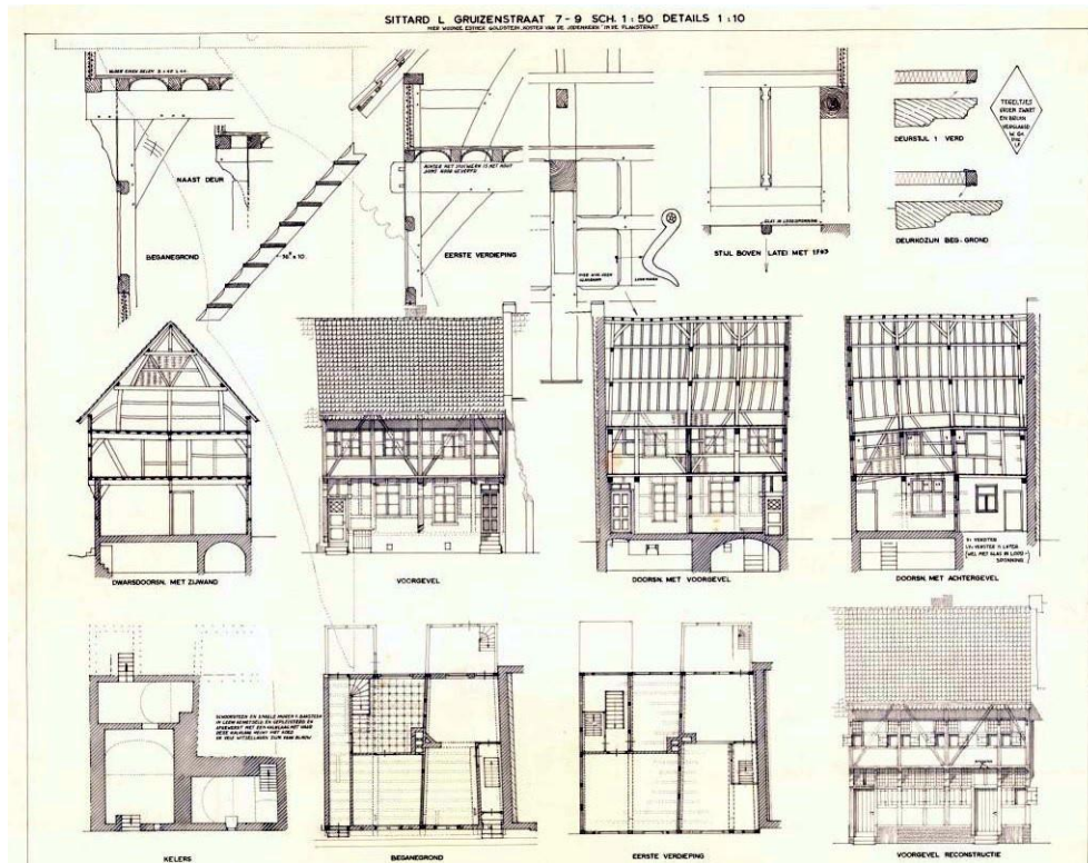
Figuur 377: Reconstructietekening van het dubbel vakwerkhuis, het huis van de koster van de Jodenkerk (Synagoge) in de Plakstraat
