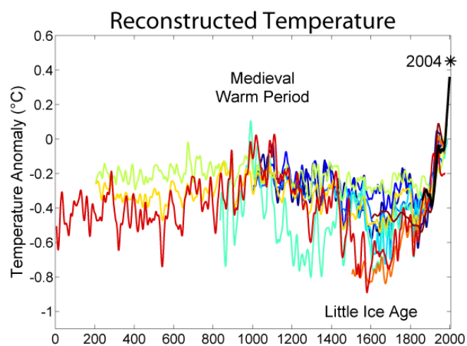
Figuur 150: Gemiddelde temperatuurafwijking in de afgelopen 2000 jaar
