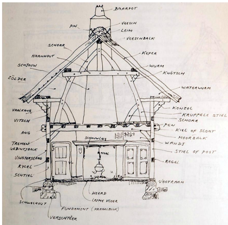
Figuur 301: Limburgse benamingen voor onderdelen van een vakwerkhuis
