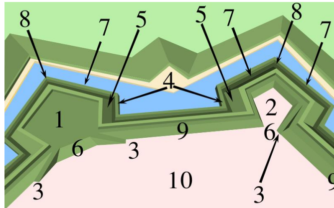
Figuur 255: Weergave van twee bastions met bijbehorende onderdelen: 1 vol bastion, 2 hol bastion, 3 april, 4 onderwal, 5 flank, 6 keel, 7 face, 8 saillant, 9 courtine en 10 terreplein
